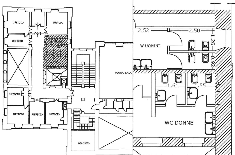
NTA POST OPERAM la 1:100 PLANIMETRIA PIANO TERZO EA DI INTERVENTO
